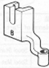
オサエアシ B Presser Foot B (φ4) 152636-001
